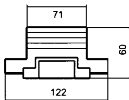
Målskisse
