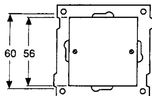
Målsskisse
