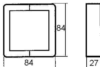
Målskisse
