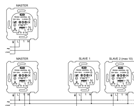
Koblingsskjema
