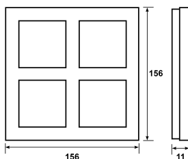
Målskisse
