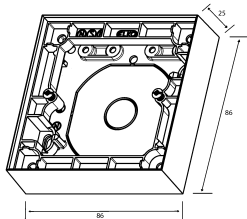
Målskisse
