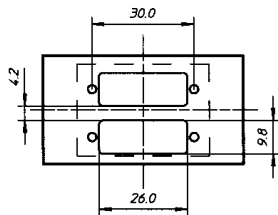
Målskisse
