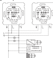
Koblingsskjema
