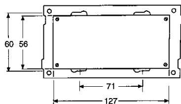
Målskisse
