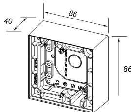
Målskisse
