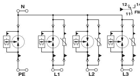
Applikasjonstegning
