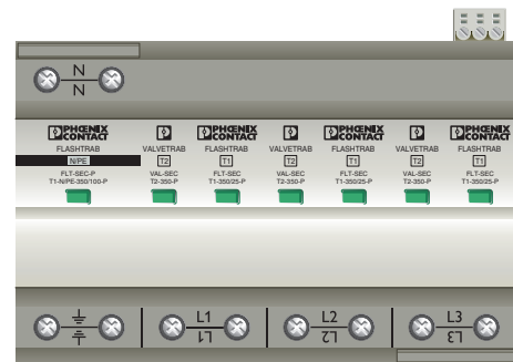
Produkttegning
