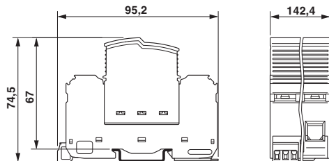
Målskisse
