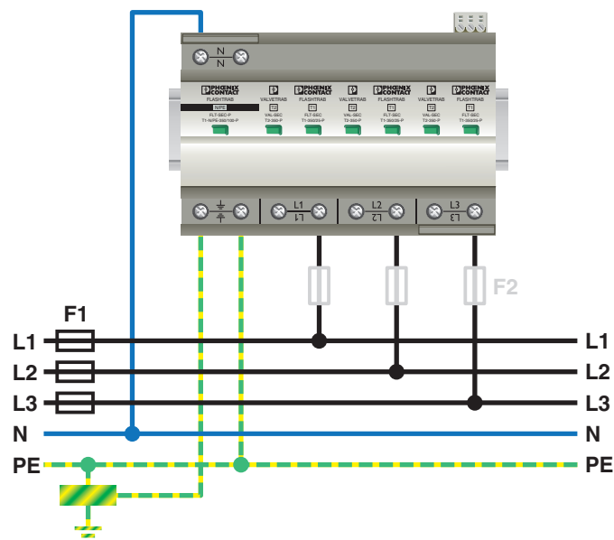
Applikasjonstegning
