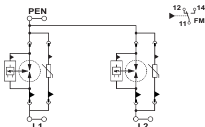
Koblingsskjema
