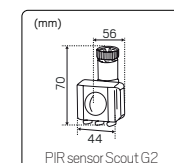
PIR sensor Scout G2
