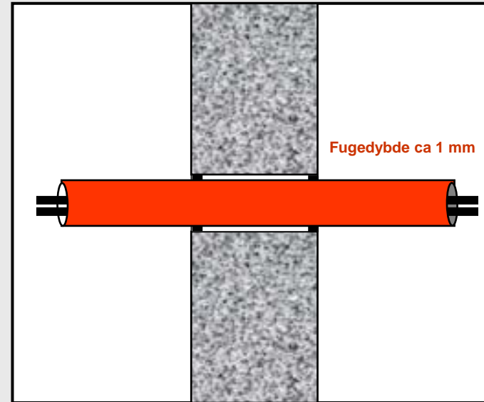
Betongvegg EI 60/EI 120
